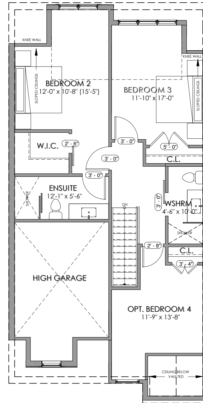
LOFT OPTION 2 851.13 SQ.FT
